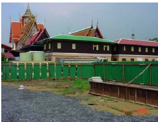
รูปที่ 4-1 ตัวอย่างรั้วกันเขตก่อสร้าง
