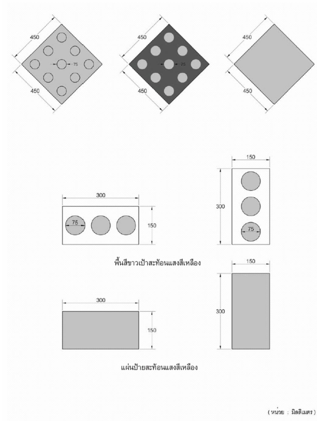
มาตรฐานเครื่องหมายเป่าสะท้อนแสง
