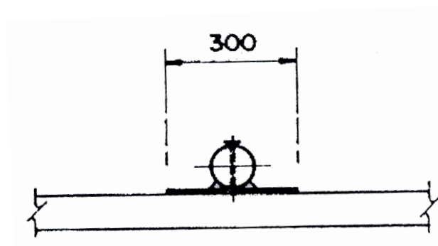
รูปที่ 7-6 การติดแผ่นเหล็กทรงด้านหลัง
