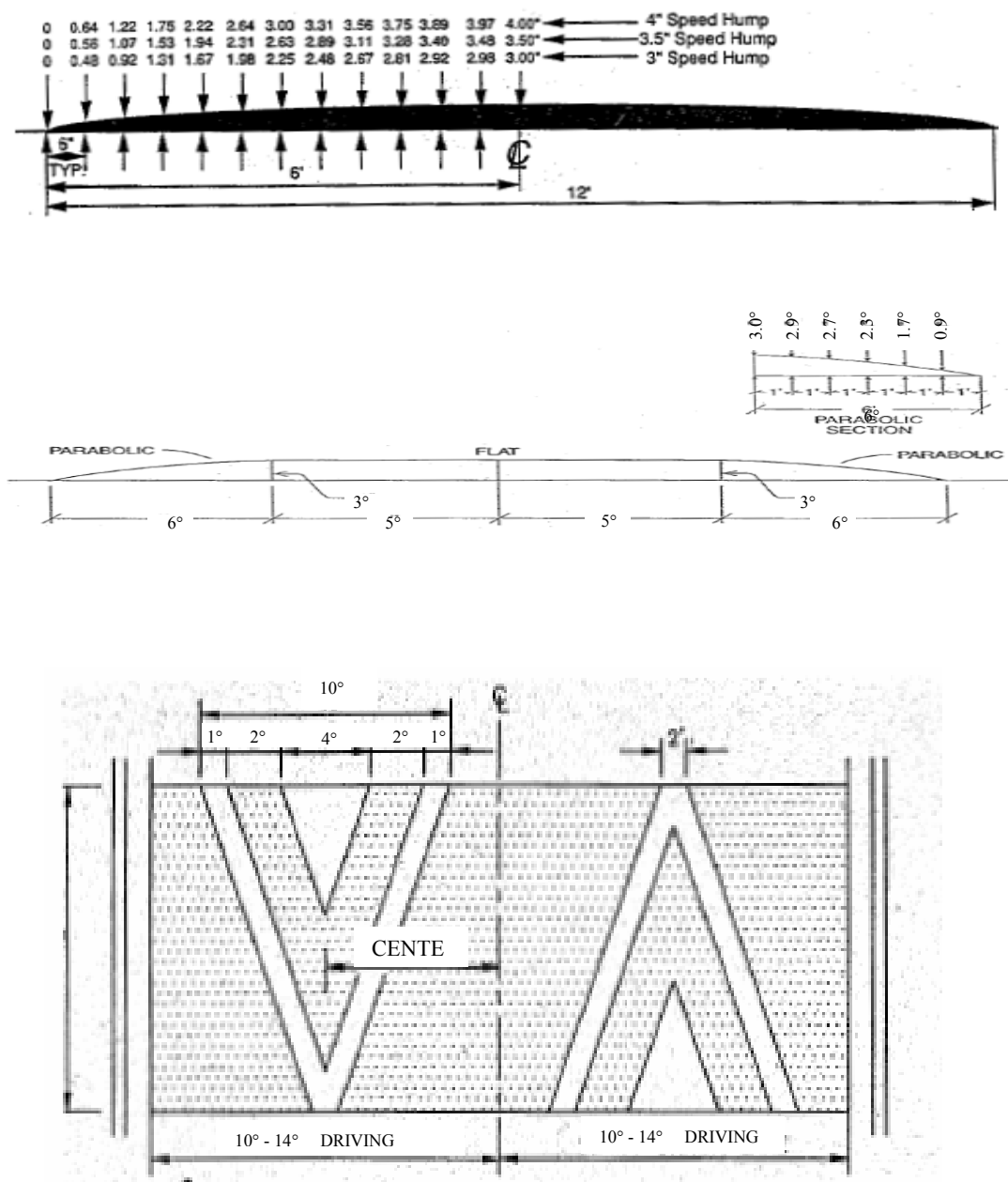
รูปที่ 6-2 ลูกเนินชะลอความเร็วแบบโค้งพาราโบลา
