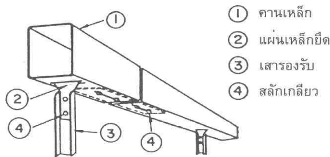
รูปที่ 7-7 ส่วนประกอบของราวกันอันตรายแบบกล่องเมื่อใช้ติดตั้งบริเวณแบ่งกันเกาะกลางถนน
