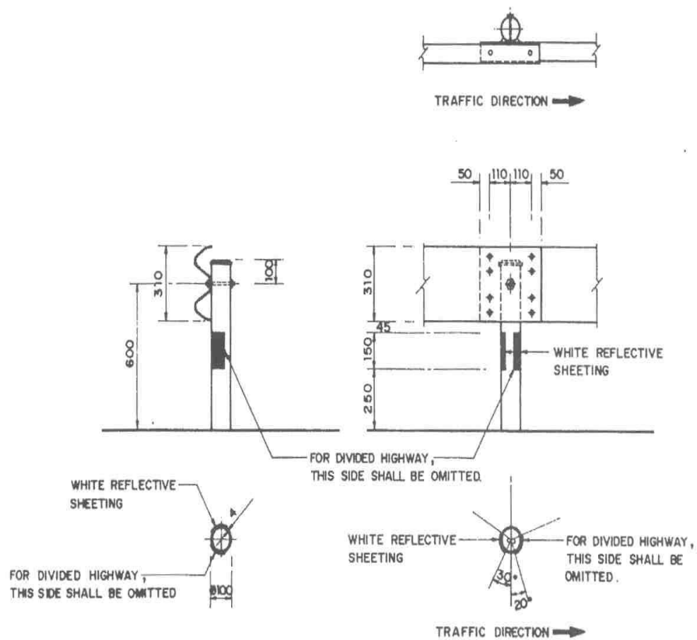
รูปที่ 7-5 เสาที่ใช้รองรับราวเหล็กลูกฟูก
